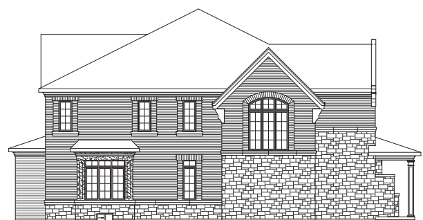
FLANKAGE ELEVATION 'B'
